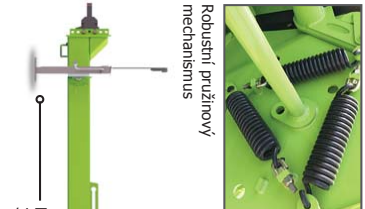
Uložení výložníku umožňuje vykládat kameny do výšky téměř dvou metrů
